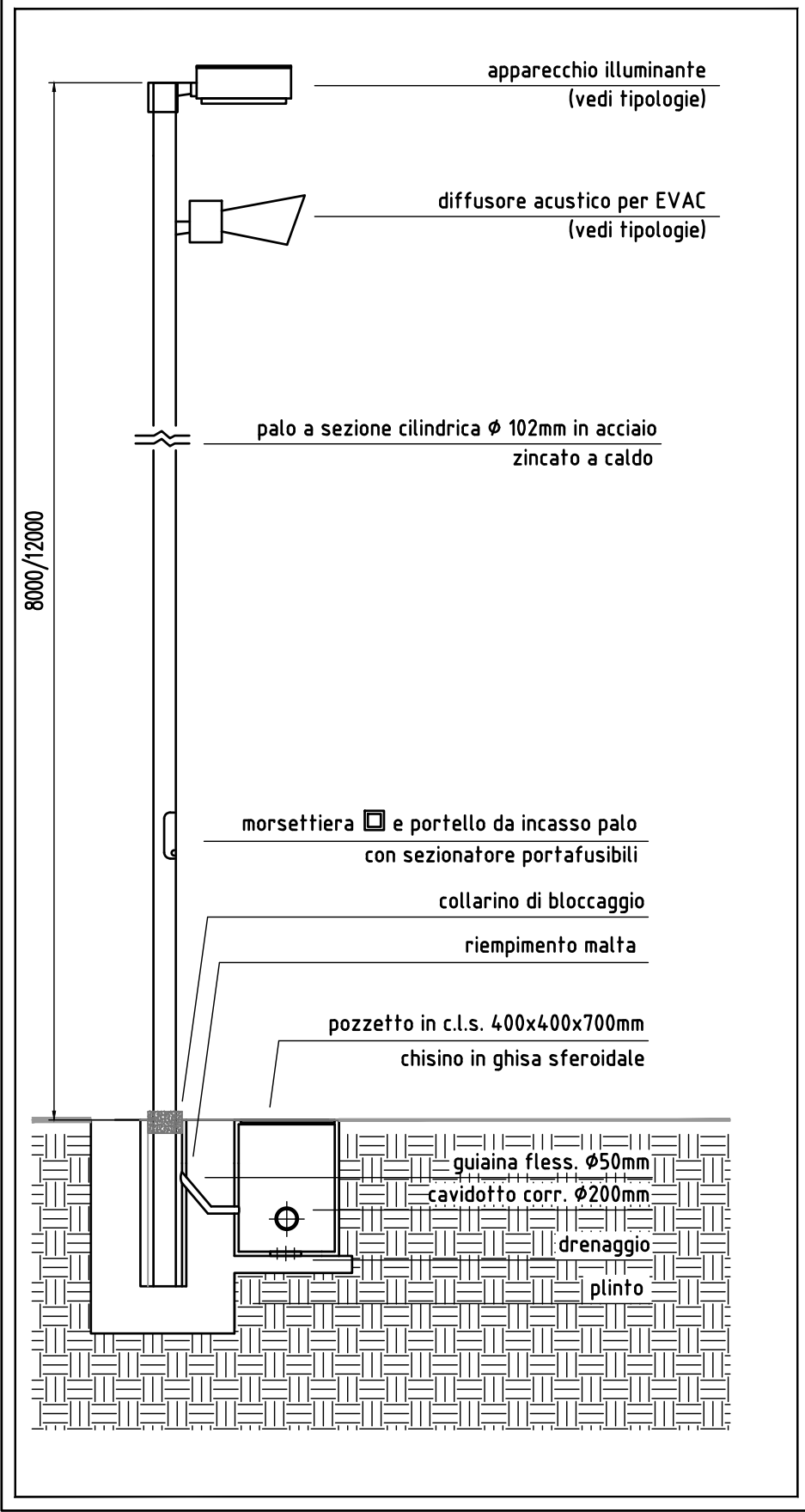
PARTICOLARE PREDISPOSIZIONE PER FUTURA INSTALLAZIONE DIFFUSORE EVAC
