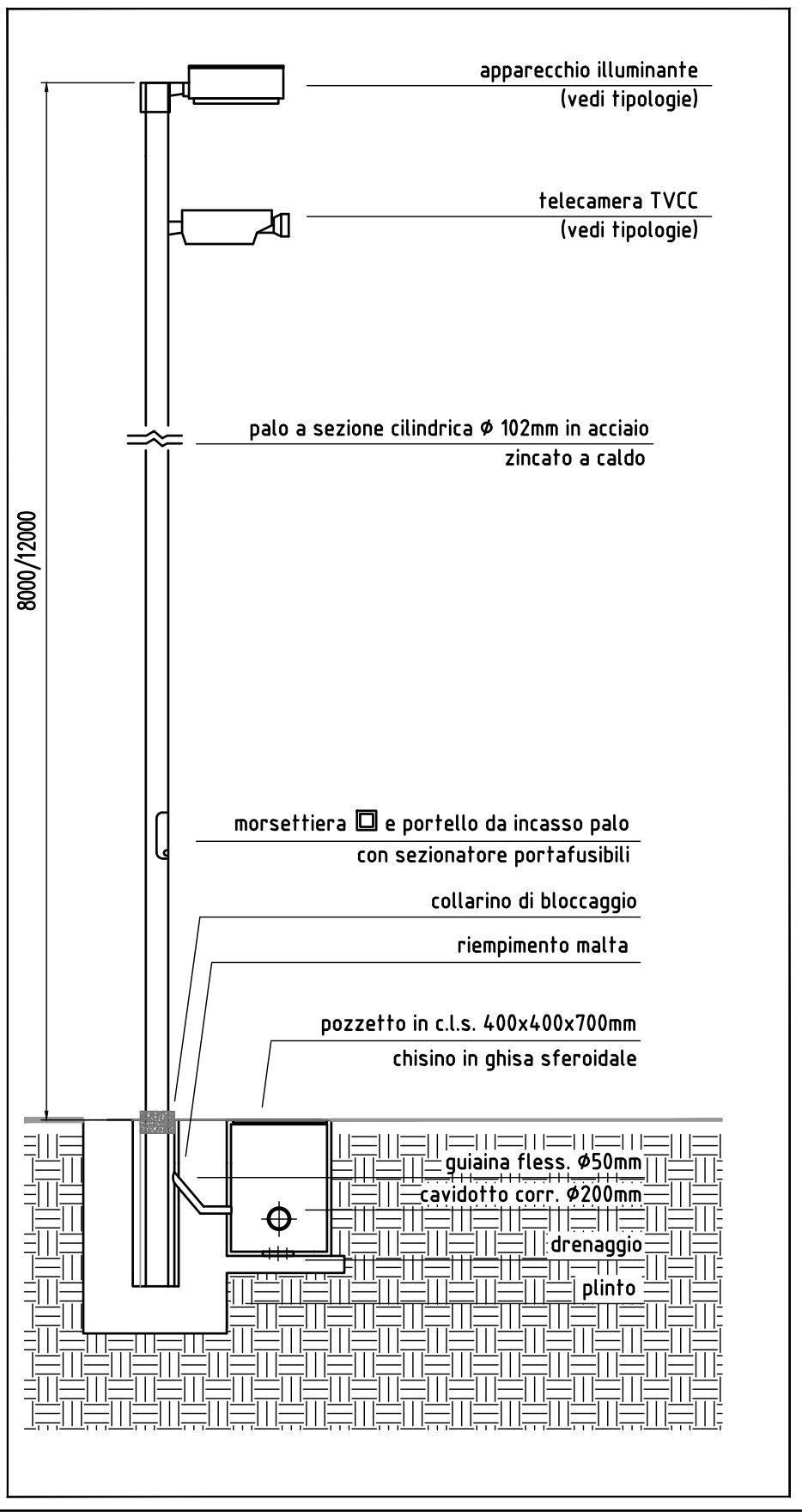
PARTICOLARE PREDISPOSIZIONE PER FUTURA INSTALLAZIONE TELECAMERA TVCC
